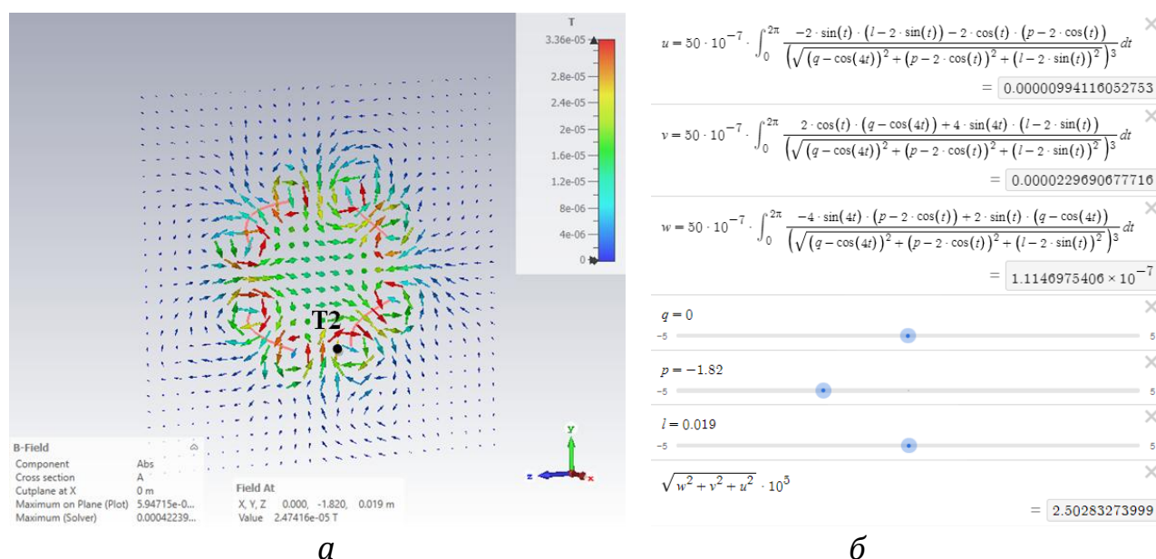
Рисунок 2 – Результаты моделирования магнитного поля: а – и расчета вектора магнитной индукции; б – по формулам (5) для точки T2 (0; -1,82; 0,019)
