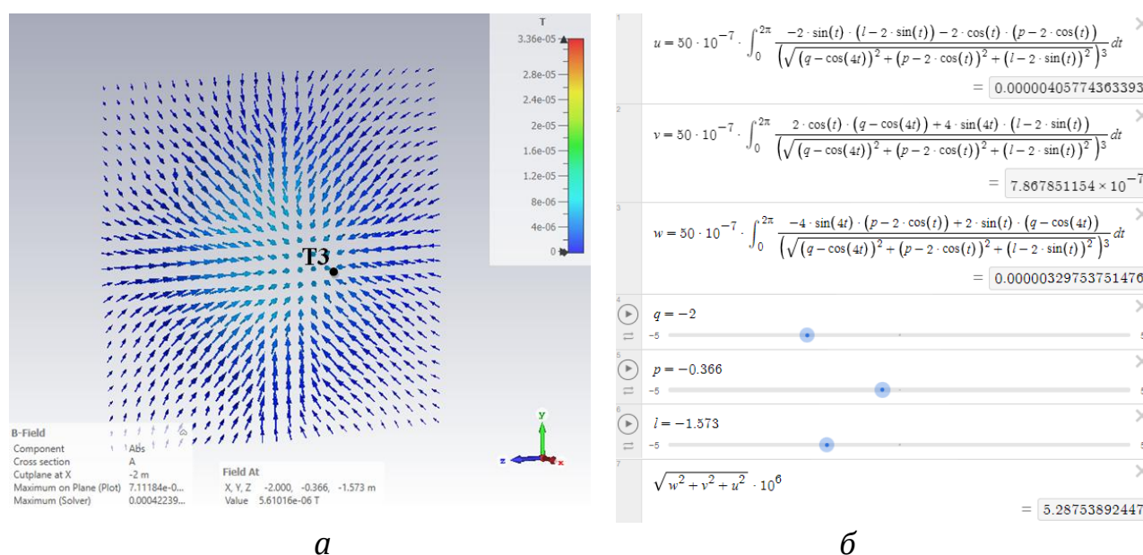
Рисунок 3 – Результаты моделирования магнитного поля: а – и расчета вектора магнитной индукции; б – по формулам (5) для точки T3 (-2; -0,366; -1,573)
