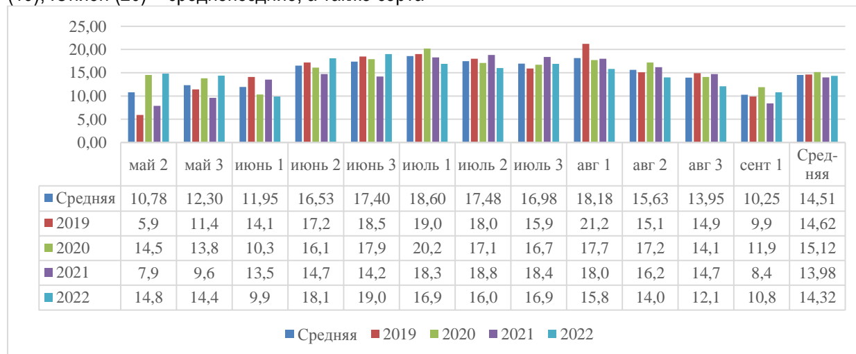
Рис. 1. Подекадные температуры воздуха Красноярской лесостепи, 2019–2022 гг., °С
