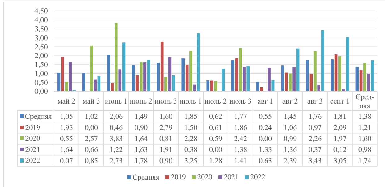
Рис. 2. Гидротермический коэффициент в Красноярской лесостепи, 2019–2022 гг.
