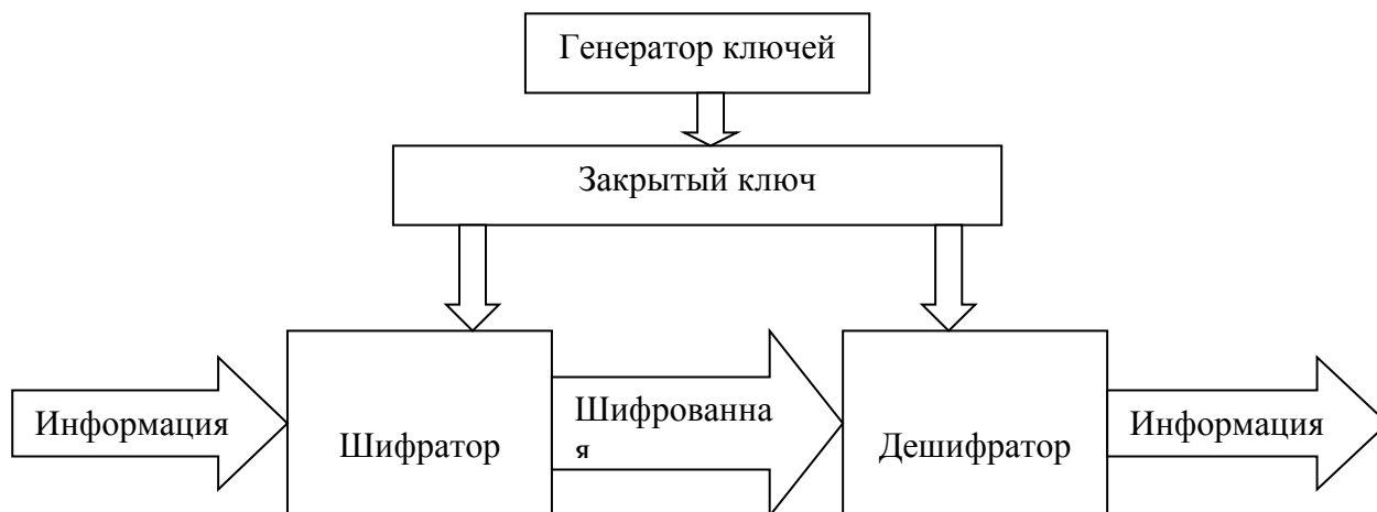
Рис. 6. Асимметричное шифрование
