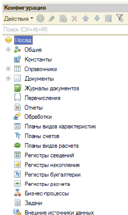
Рисунок 7. Дерево конфигурации
