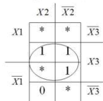
Функция f c
