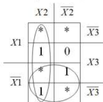
Функция f b
