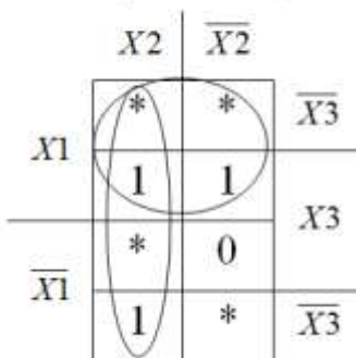
Функция f a
