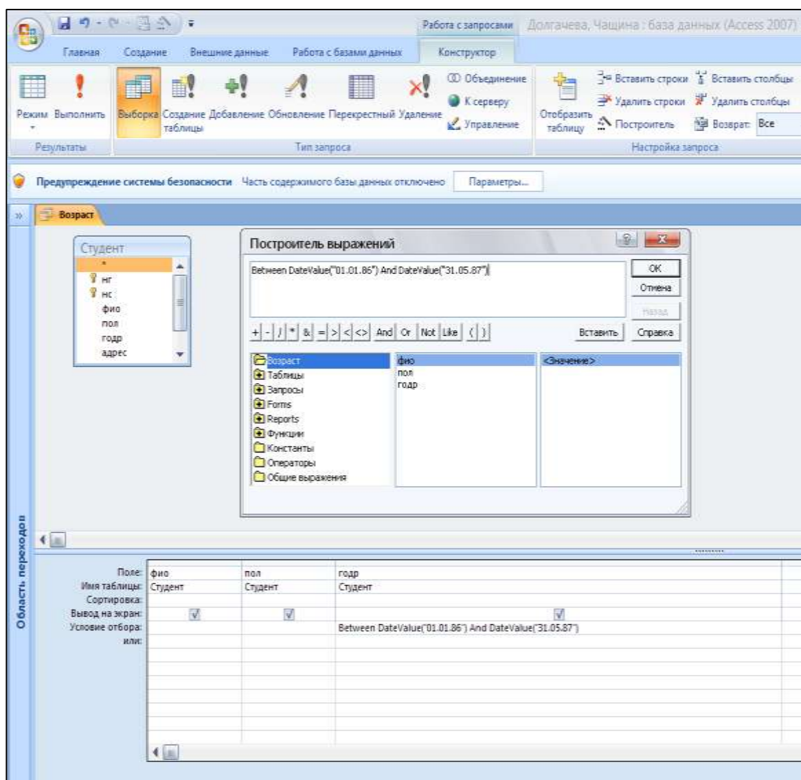
Рис. 54. Выполнение запроса 1
