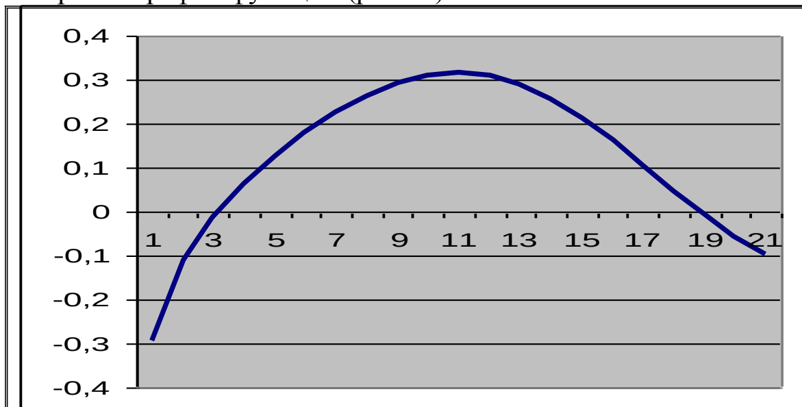
Рис. 13. График функции
