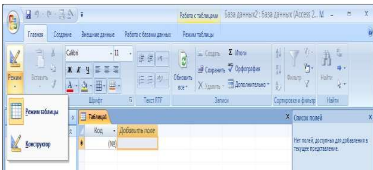
Рис. 49. Режим таблицы
