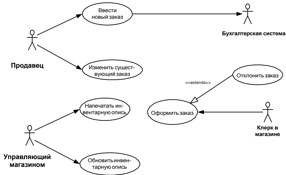
Рис. 1. Диаграмма вариантов использования для системы обработки заказов
