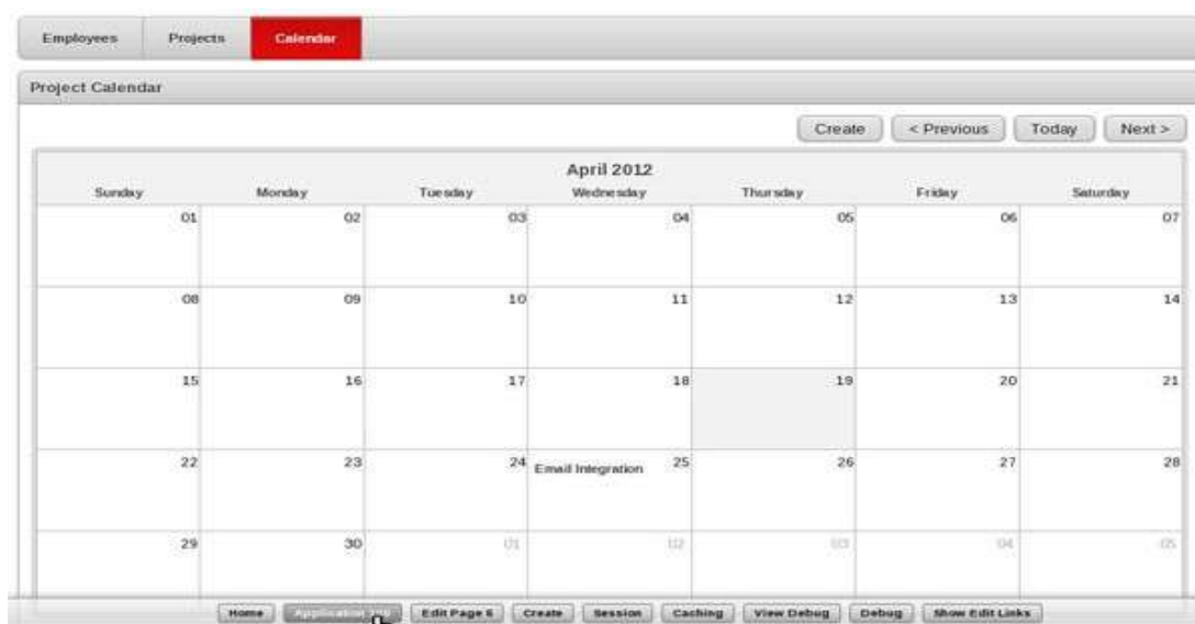
Рисунок 20: Календарь
