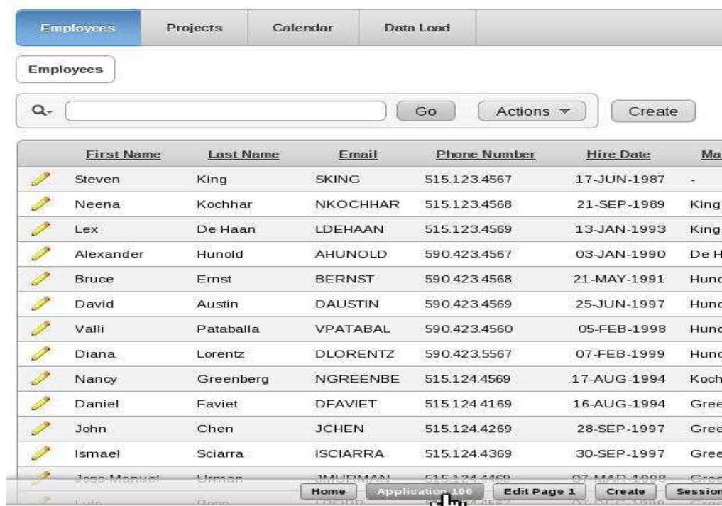
Рисунок 24: Новый стиль
