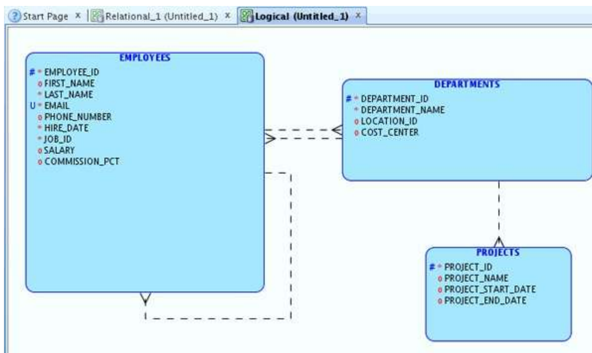
Рисунок 6: Логическая модель
