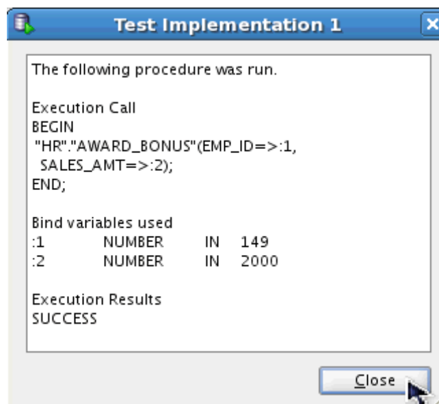
Рисунок 16: Окончание тестирования
