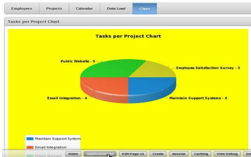
Рисунок 25: Диаграмма
