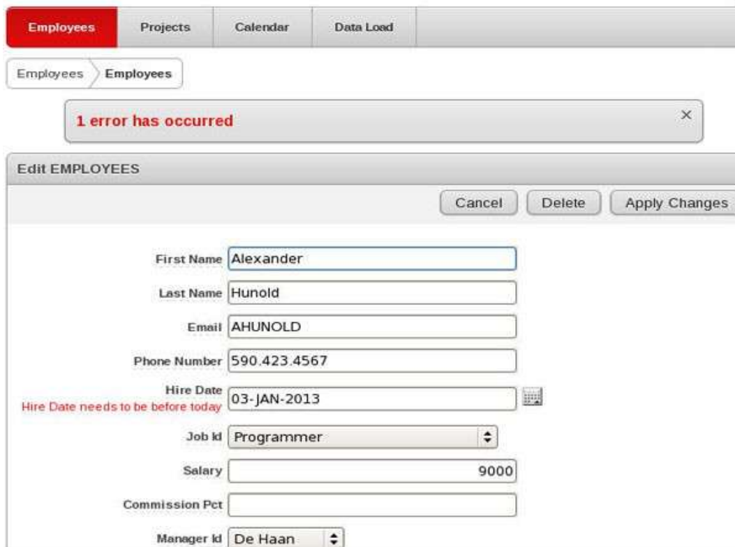
Рисунок 23: Проверка
