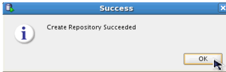
Рисунок 15: Репозитарий создан
