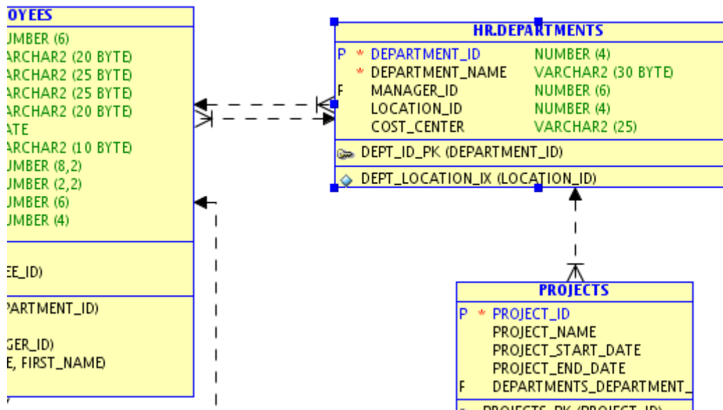
Рисунок 5: Новый столбец
