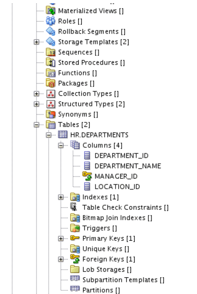
Рисунок 2: Физическая модель
