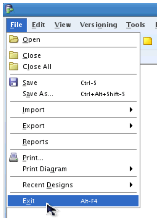
Рисунок 9: Выход
