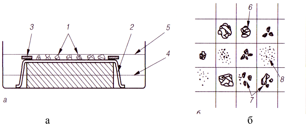
Рисунок 3. Схема опыта по определению водопрочности агрегатов а – приспособление для увлажнения агрегатов; б - участок фильтра с агрегатами:
