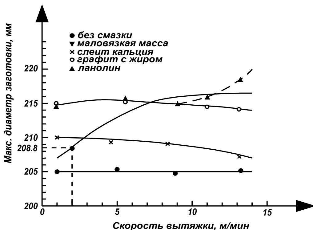
Рисунок 6.1 – Скорость вытяжки, м/мин
