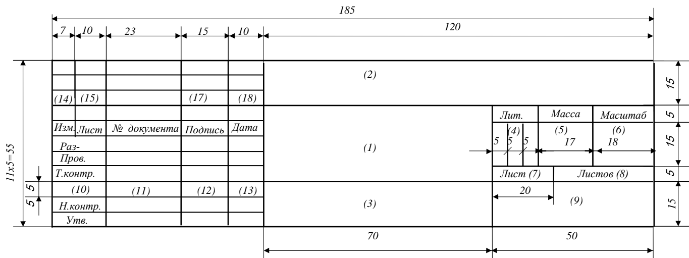
Форма 2 (ГОСТ 2.104) – Основная надпись для заглавных листов текстовых конструкторских документов
