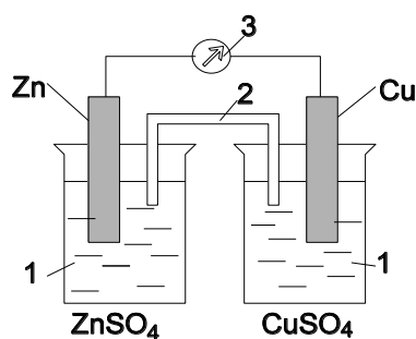
Рисунок 9.1 – Медно—цинковый гальванический элемент
