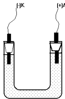
Рис. 9.2. Схема установки для проведения электролиза.
