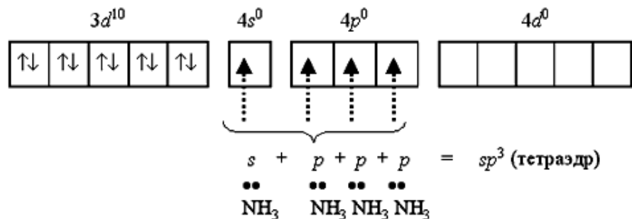
Рис. 7.1. Схема образования катиона [\text{Zn}(\text{NH}_3)_4]^{2+}
