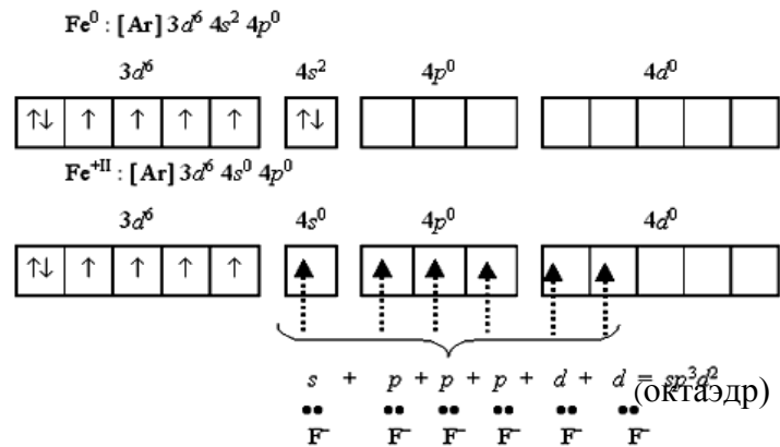
Рис. 7.2. Схема образования аниона [\text{FeF}_6]^{4-}
