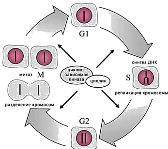
Рисунок 12 – Клеточный цикл
