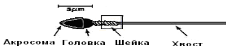
Рисунок 18 – Строение сперматозоида
