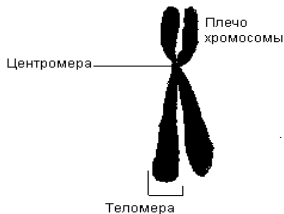
Рисунок 8 – Строение хромосомы
