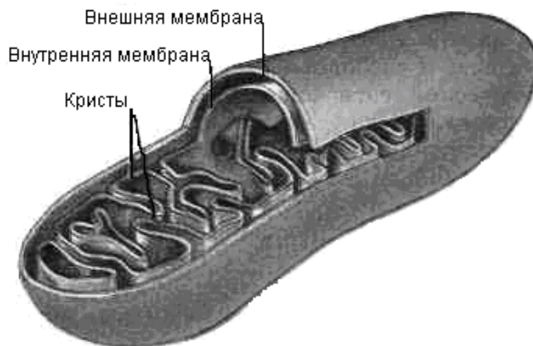
Рисунок 5 – Строение митохондрии
