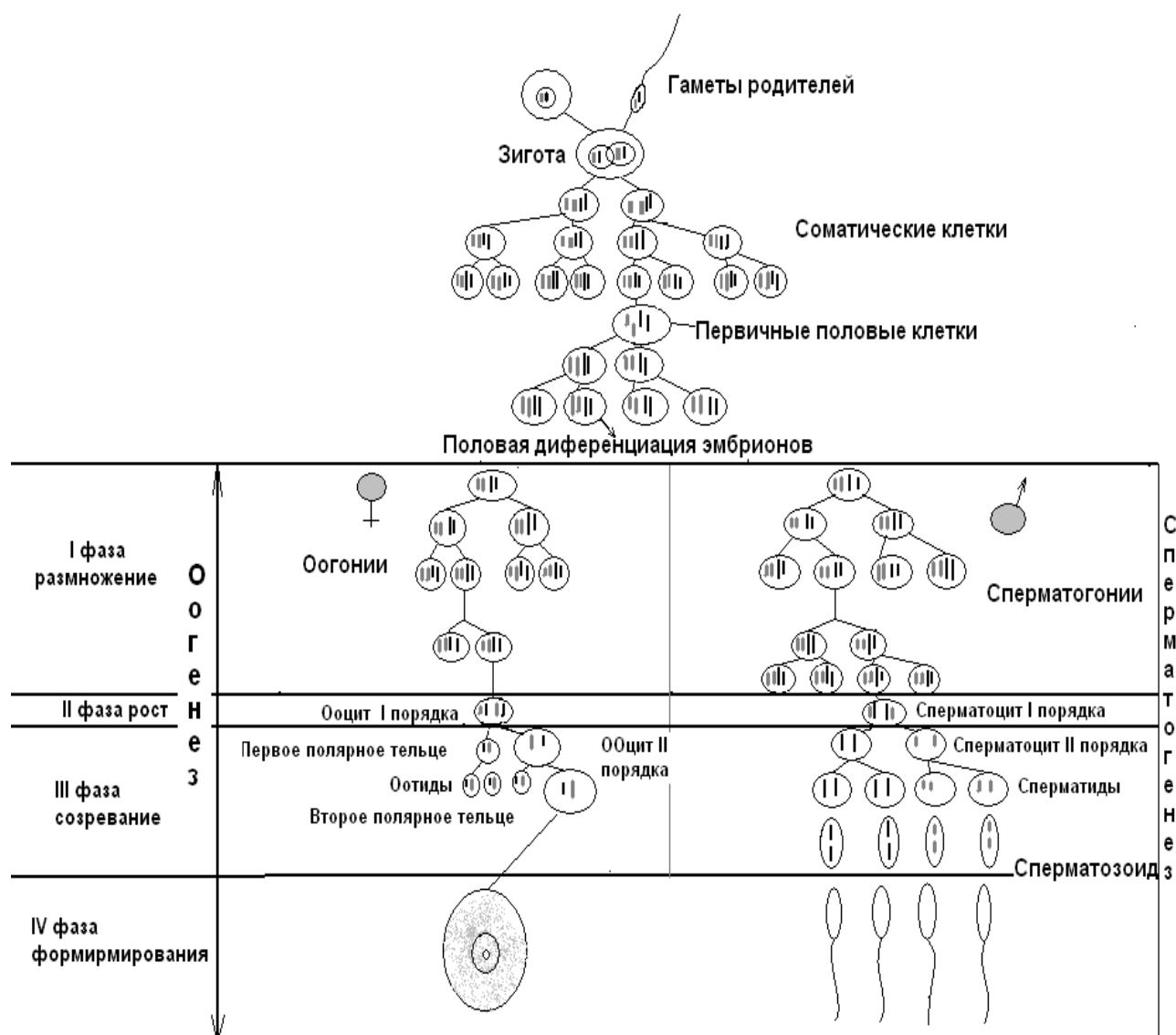
Рисунок 16 – Схема гаметогенеза [1]
