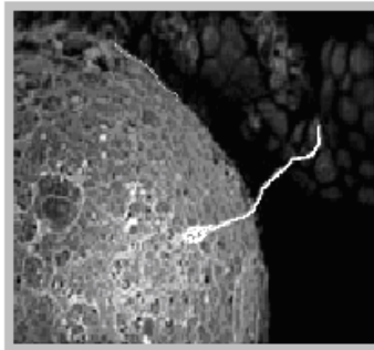
Оплодотворяемая яйцеклетка
