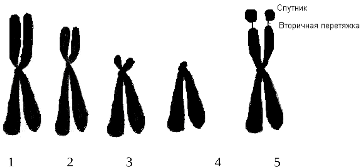
Рисунок 9 – Виды хромосом:
