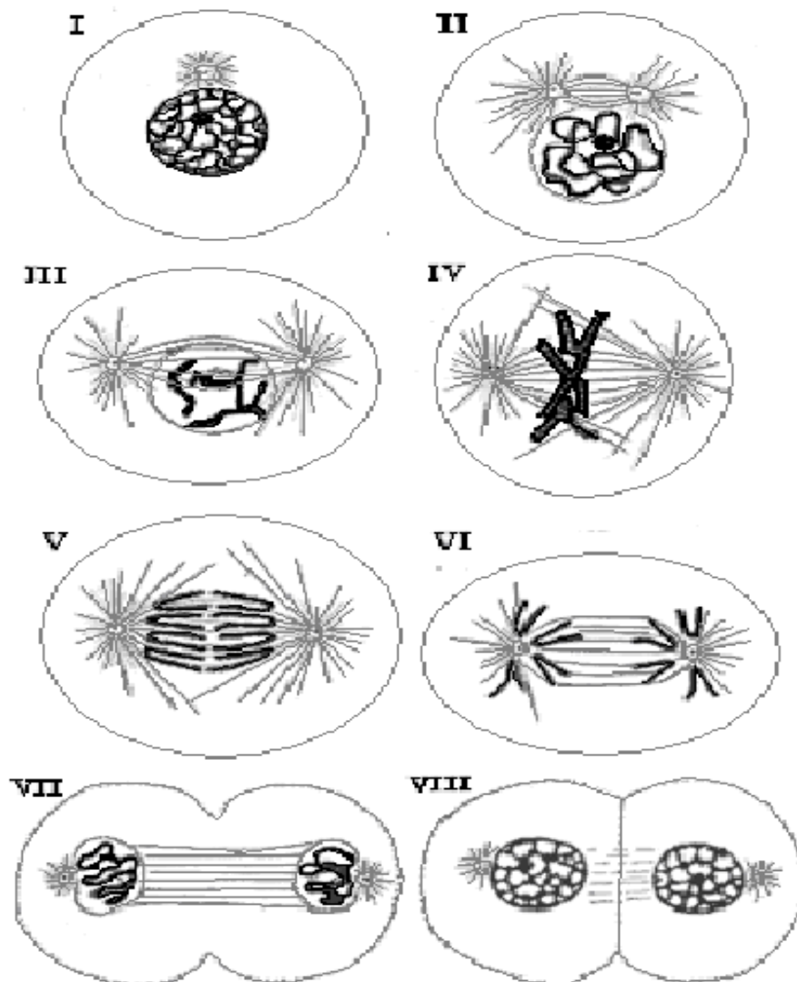
Рисунок 13 – Фазы митоза:
