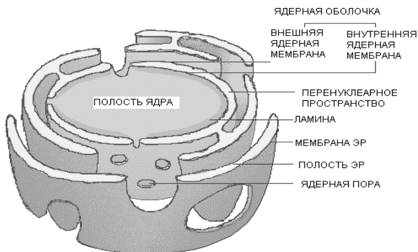
Рисунок 4 – Строение ядра
