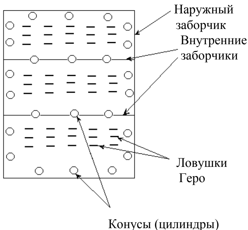
Рисунок 1 – Обустройство огороженной площадки конусами (цилиндрами) и плашками Геро (по Соколову и др., 1974)
