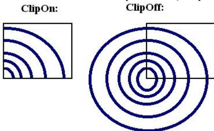
Рис. 4.1. Отсечка изображения в окне Uses Graph,CRT;
