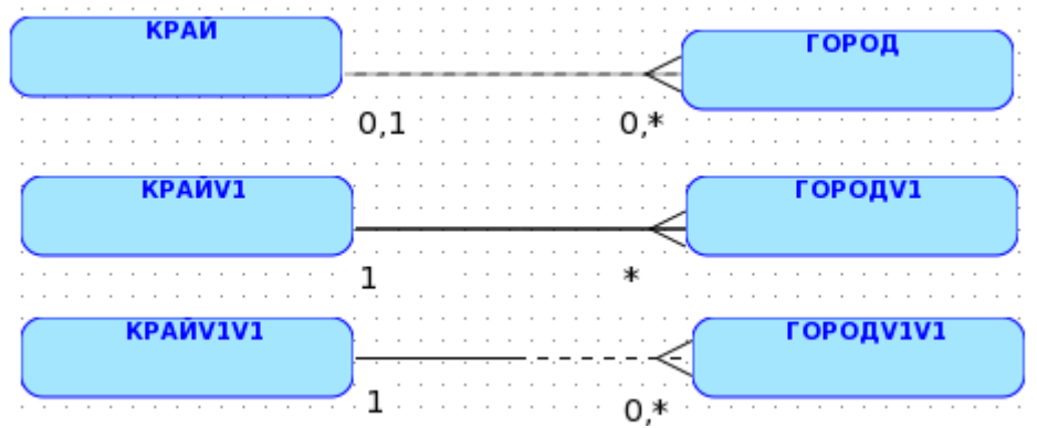
Рис. 6 Связь один-ко-многим в нотации Баркера
