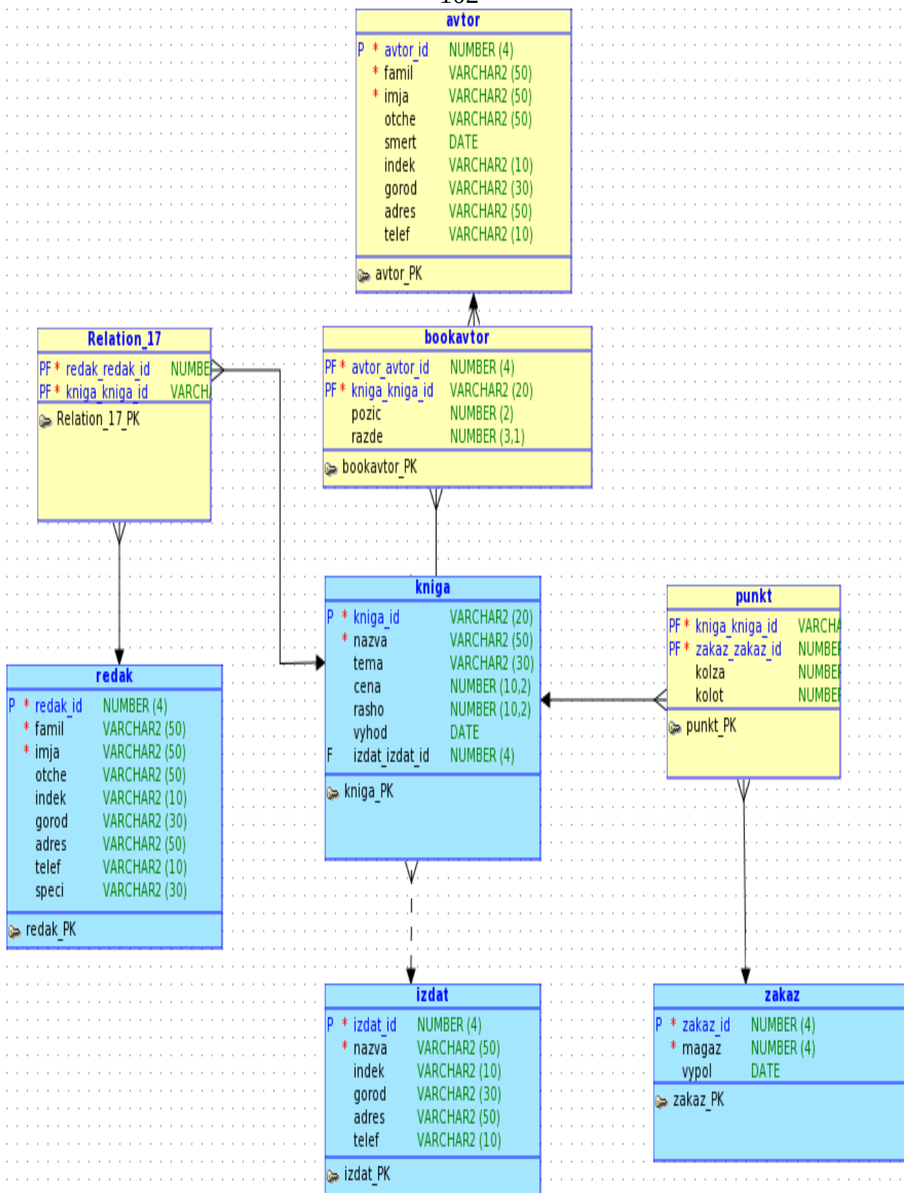
Рис. 21: Реляционная модель
