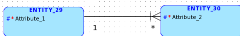
Рис. 9 Идентифицирующая связь в нотации Баркера
