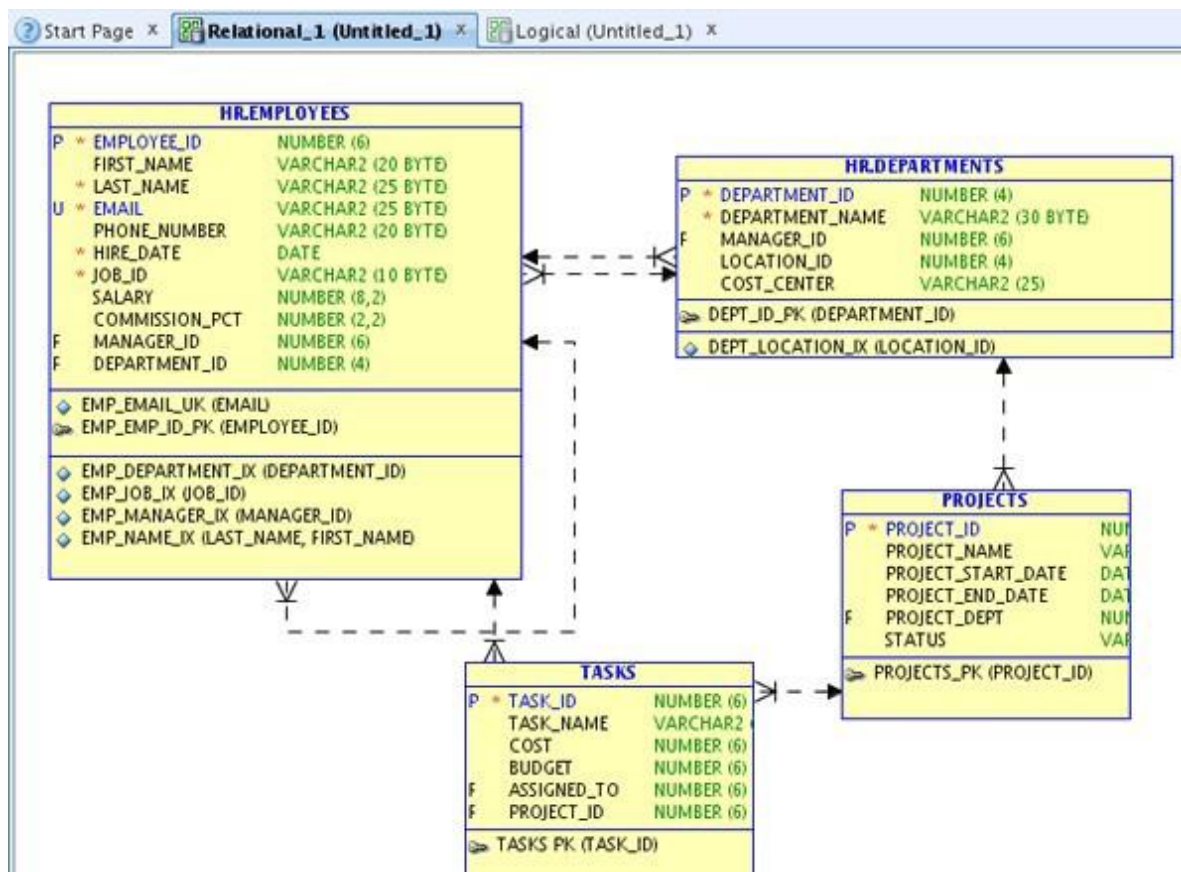
Рисунок 8: Реляционная модель после синхронизации
