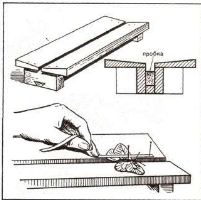
Рис. 5. Расправилка
