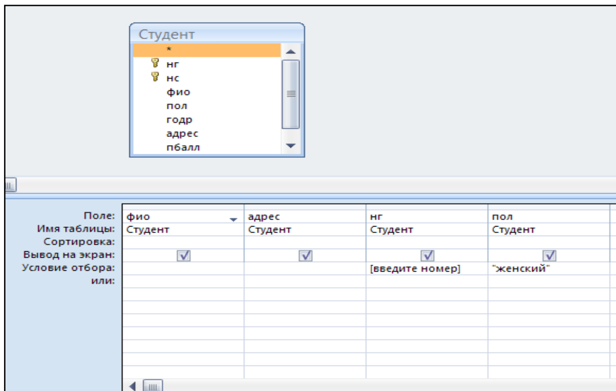
Рис. 53. Бланк запроса с параметром (запрос № 2)
