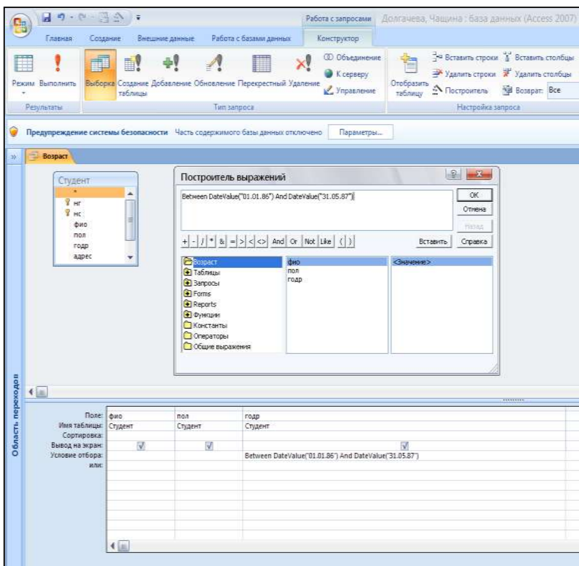
Рис. 54. Выполнение запроса 1
