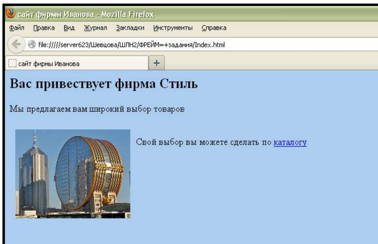
Рис. 85. Просмотр web-страницы
