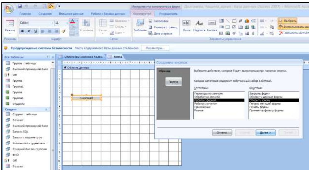
Рис. 64. Конструктор форм
