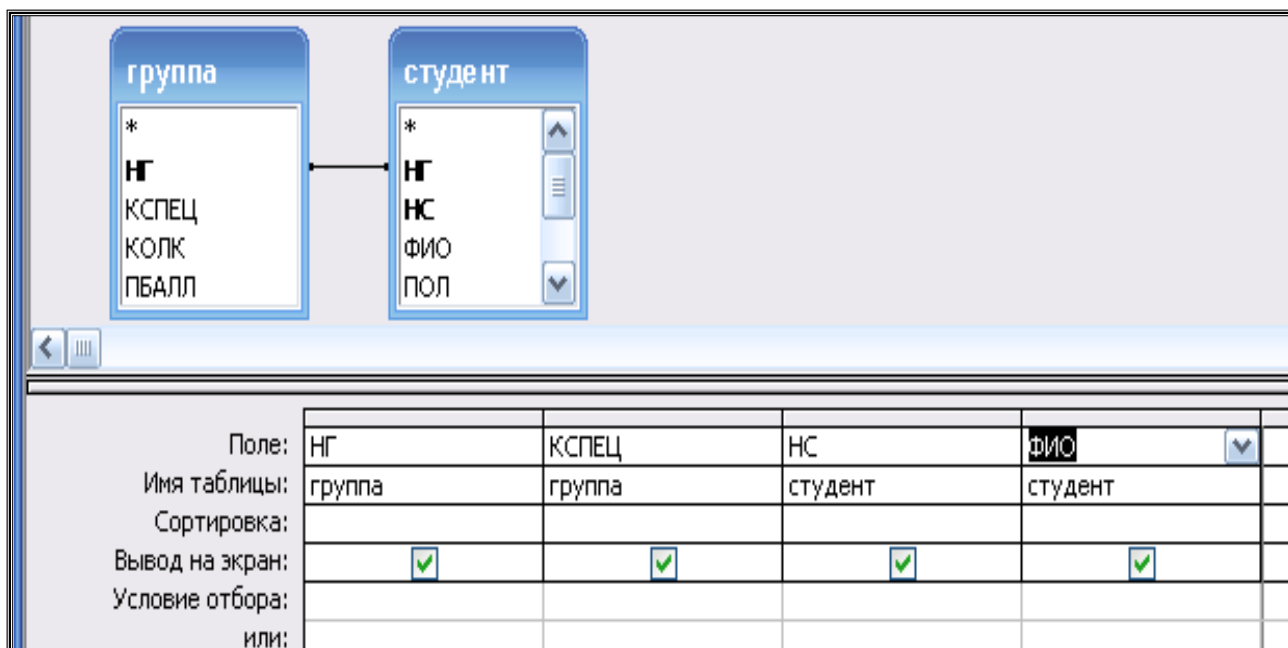
Рис. 58. Выбор готовых полей
