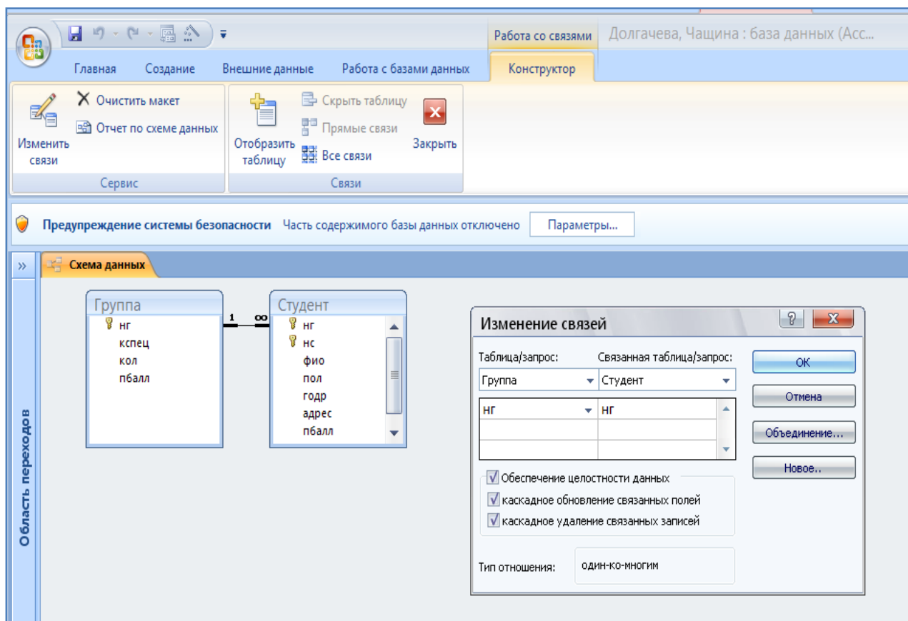
Рис. 52. Окно «Схема данных»
