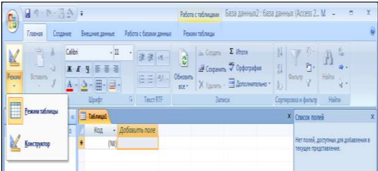
Рис. 49. Режим таблицы
