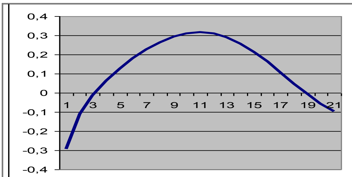
Рис. 13. График функции
