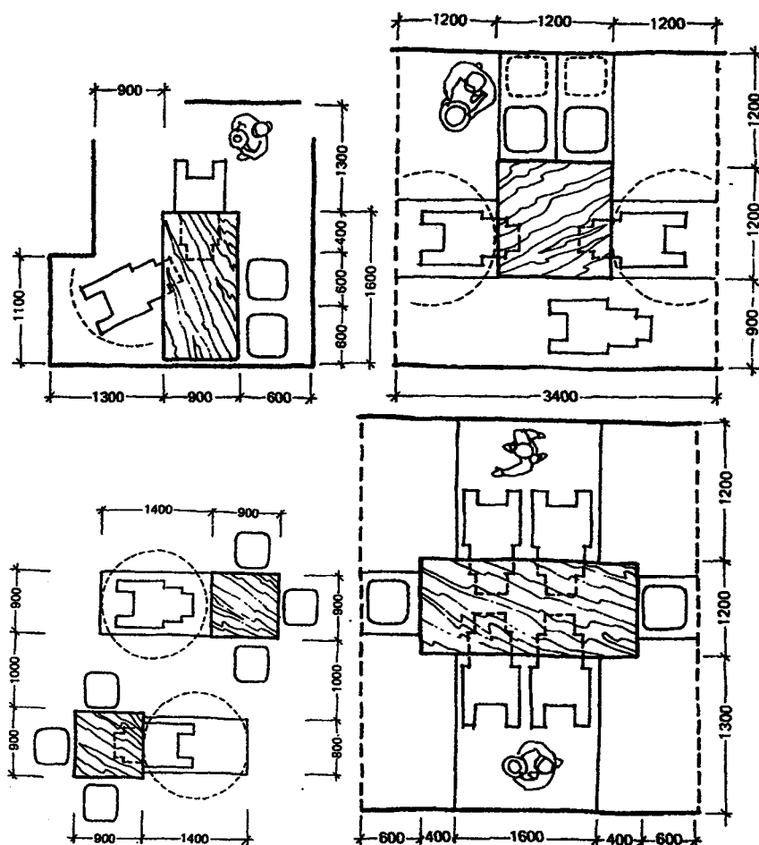
Рис. 46. Оборудование обеденных залов столовых, адаптируемых к посещению людей с ограниченными возможностями
