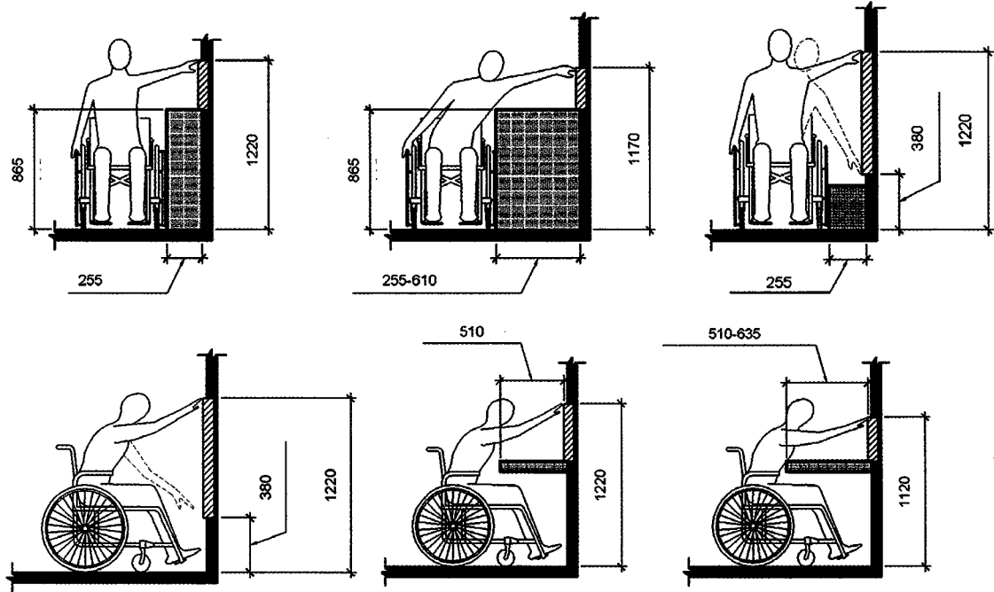
Рис. 30. Параметры доступа к оборудованию
