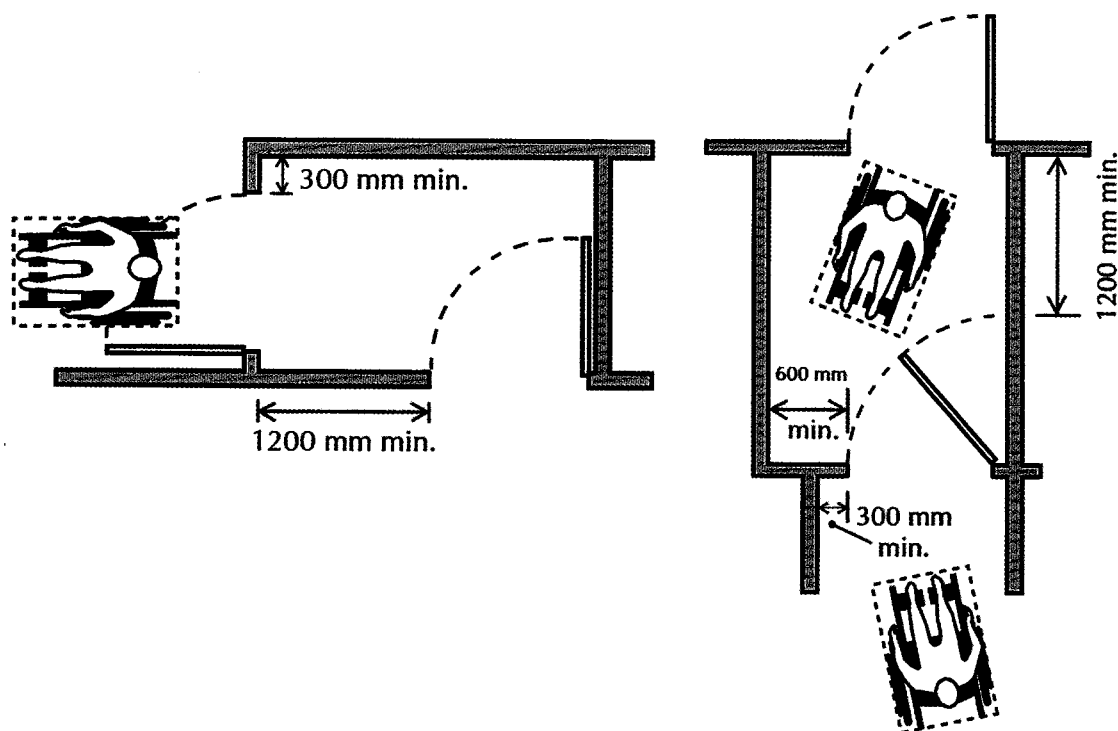
Рис. 14. Рекомендуемое размещение входных дверей
