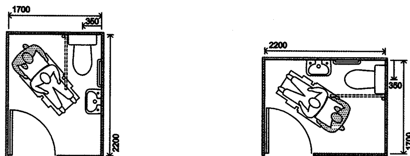
Рис. 36.2. Схемы пересадки и требуемые габариты кабин
