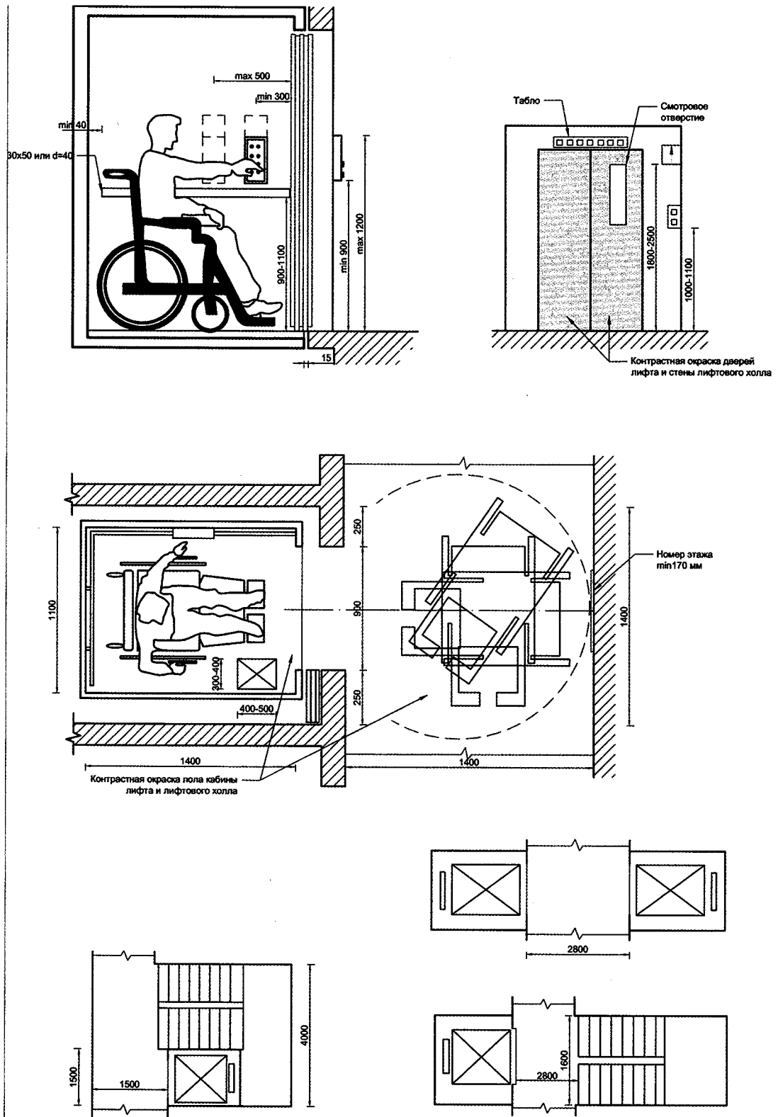
Рис. 19 Оборудование лифта
