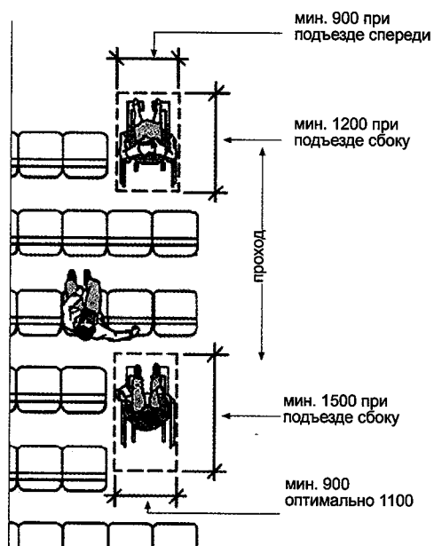
Рис. 52. Габариты мест для кресел-колясок. Скругление углов стен
