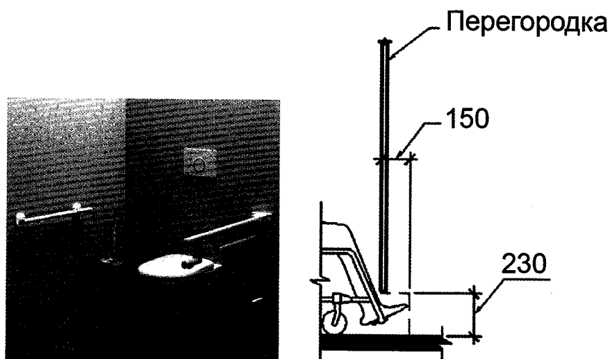
Рис. 37. Пример оборудования санузла опорными поручнями, установка санитарных перегородок
