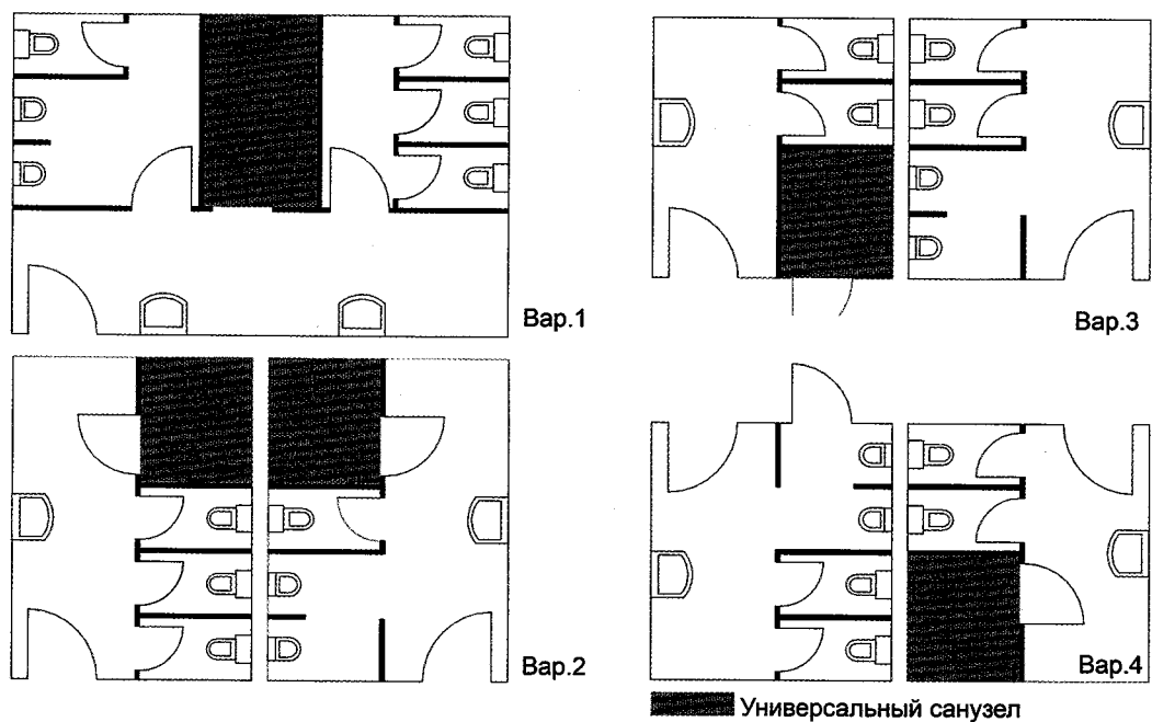
Рис. 36.1. Схемы пересадки и требуемые габариты кабин
