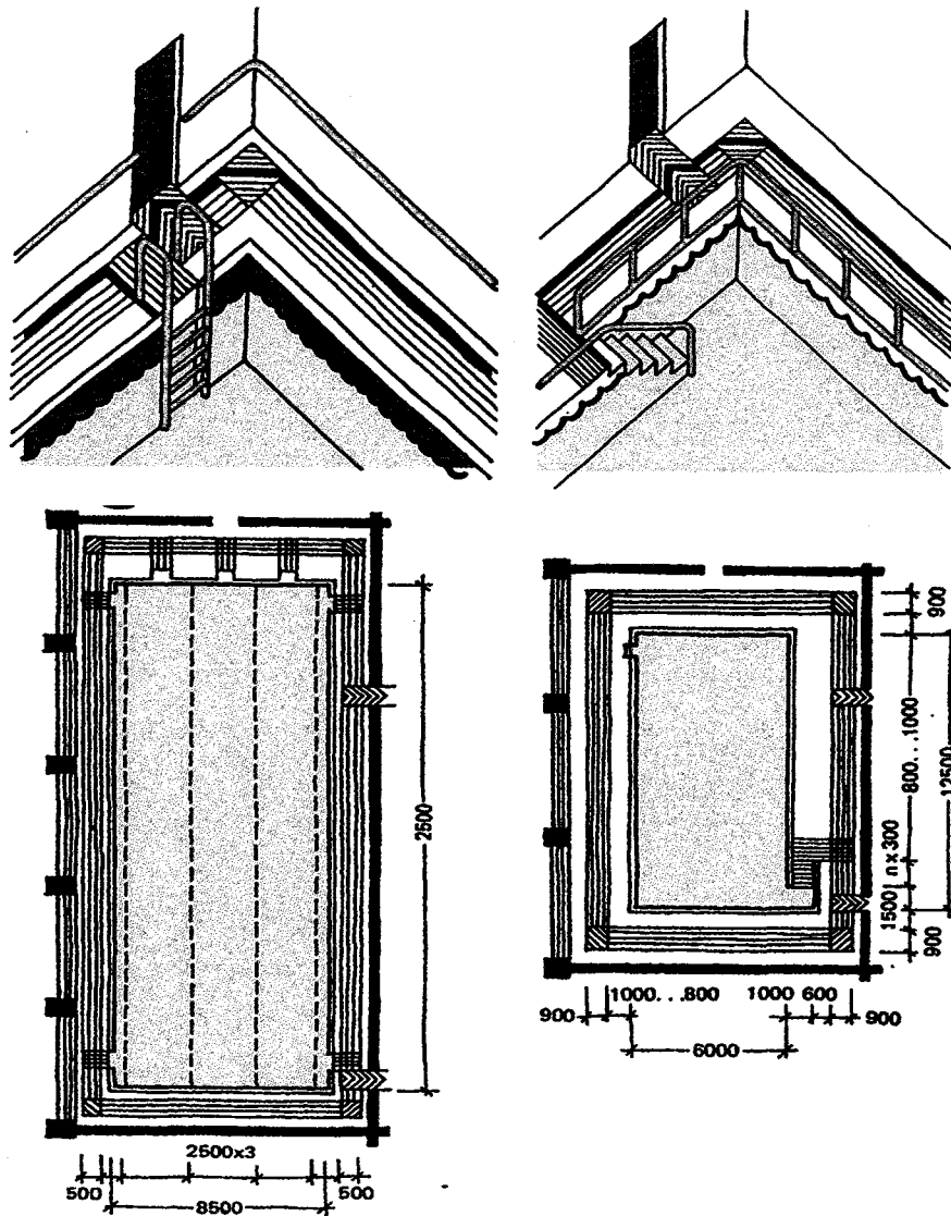
Рис. 48. Оборудование бассейнов обходными дорожками с фактурной поверхностью
