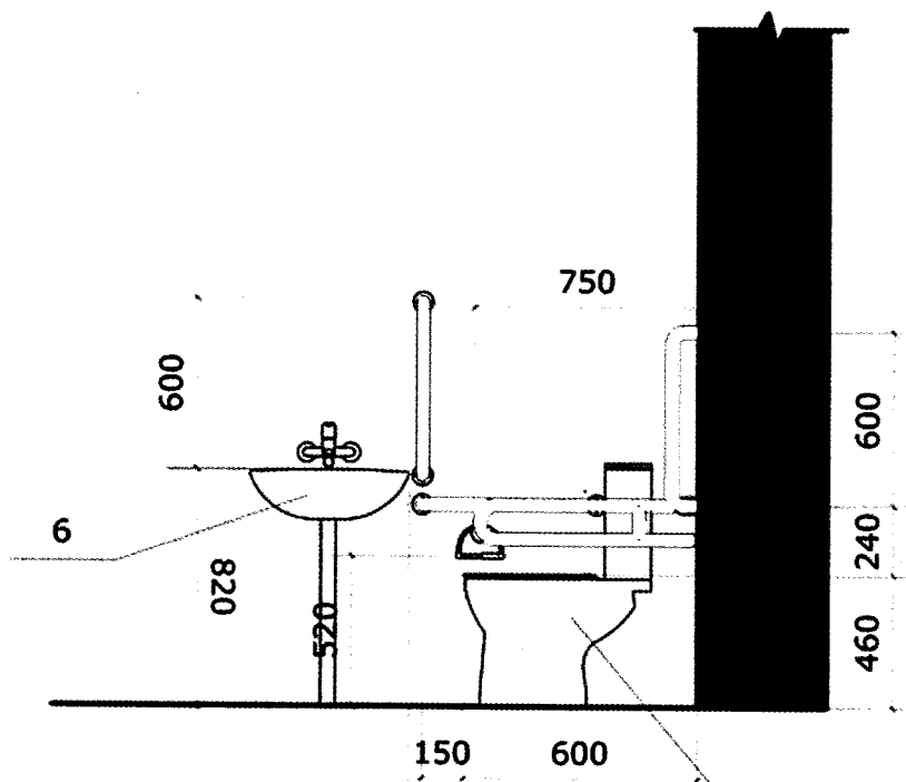
Рис. 42. Пример оборудования санузла поручнями контрастного цвета
