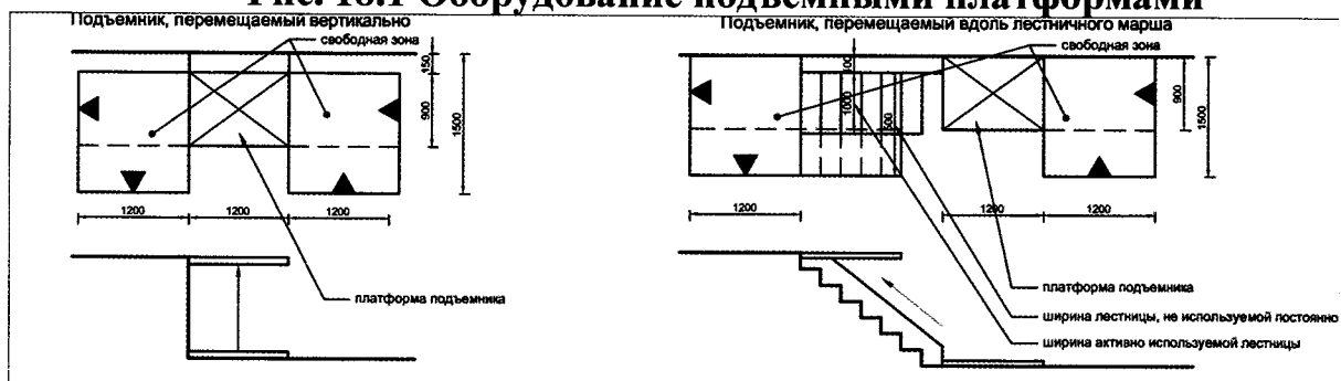
Рис. 18.1 Оборудование подъемными платформами
