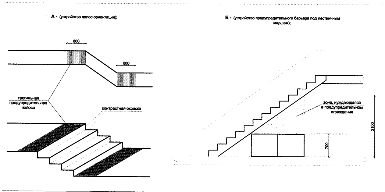
Рис. 23 Полосы ориентации, контрастная окраска и тактильные предупредительные полосы
