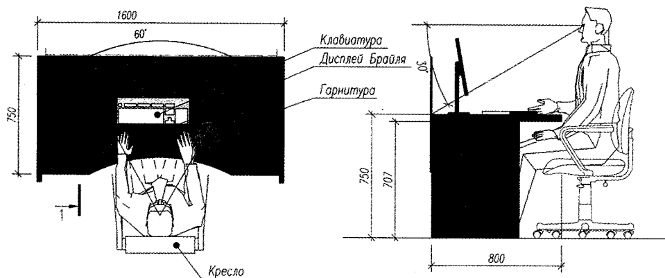
Рис. 33. Параметры учебного компьютерного места учащегося
