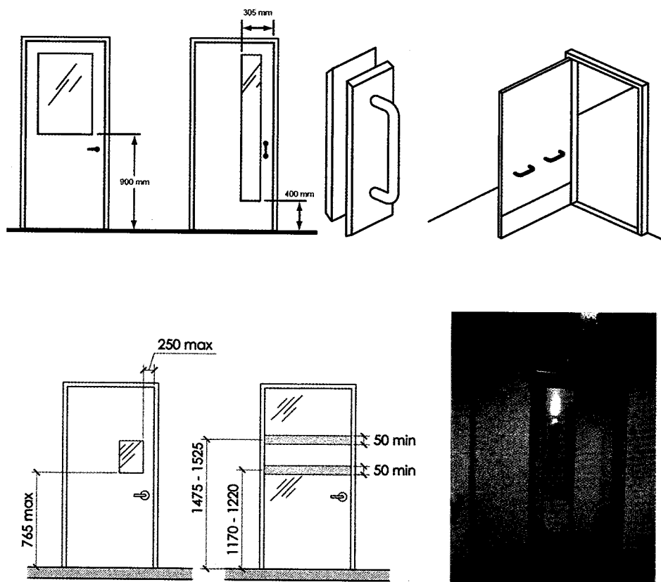
Рис. 41. Остекленные проемы дверей и маркировка
