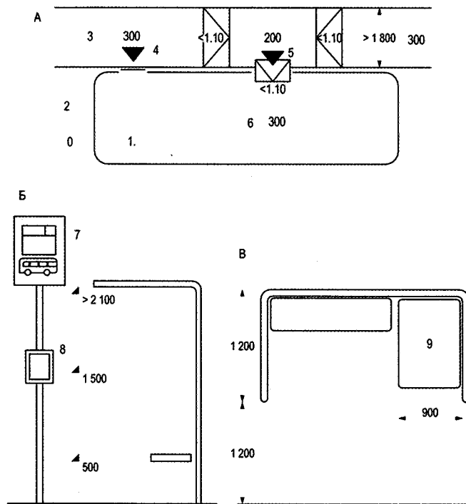
Рис. 6. Примеры оборудования автобусных остановок
