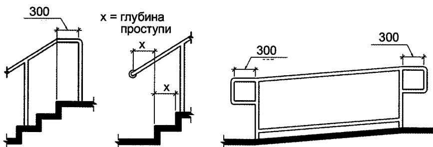
Рис. 25.1. Завершение поручней. Тактильные указатели
