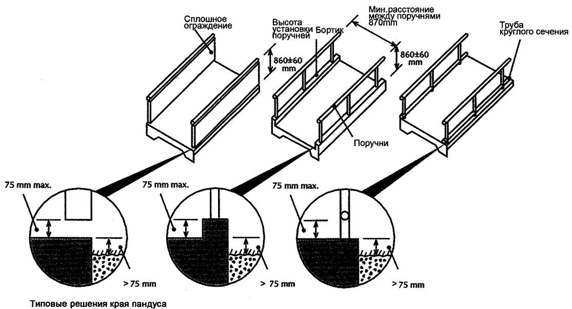
Рис. 28. Защита от соскальзывания на пандусах
