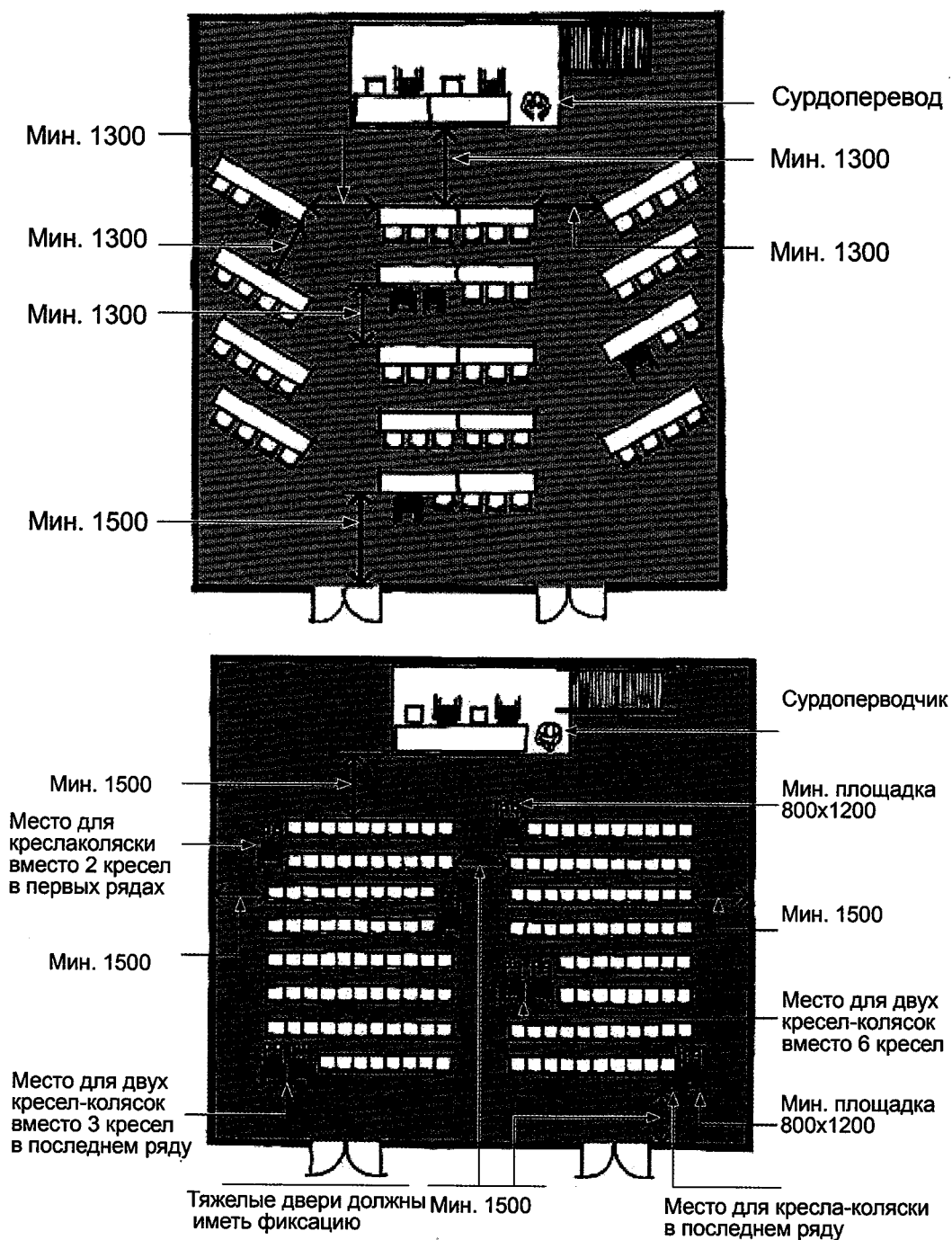
Рис. 50. Оборудование зрительных залов
