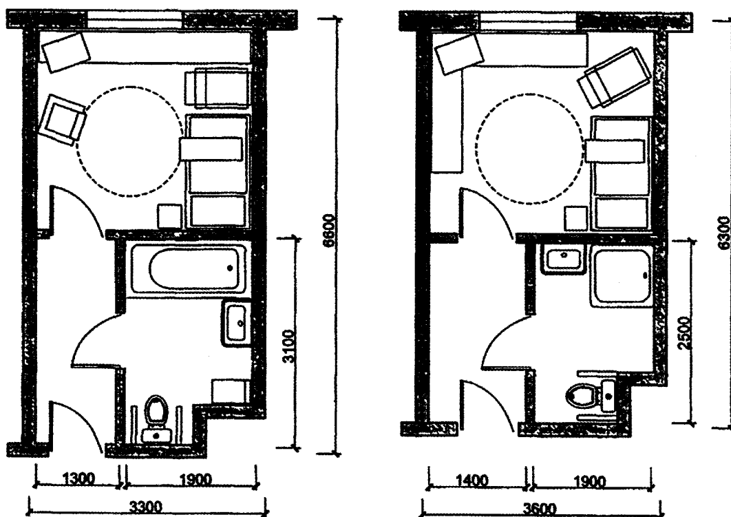
Рис. 34. Оборудование комнаты, для проживания одного человека с ограниченными возможностями
