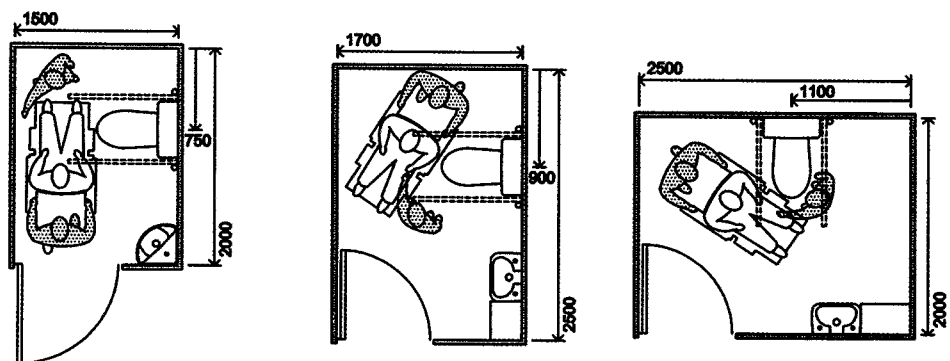
Рис. 36.1. Схемы пересадки и требуемые габариты кабин
