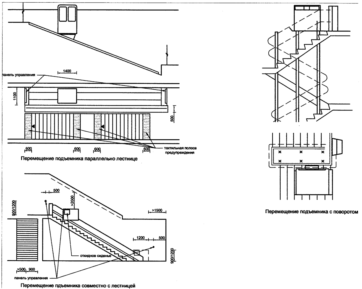
Рис. 18.3 Оборудование подъемными платформами
