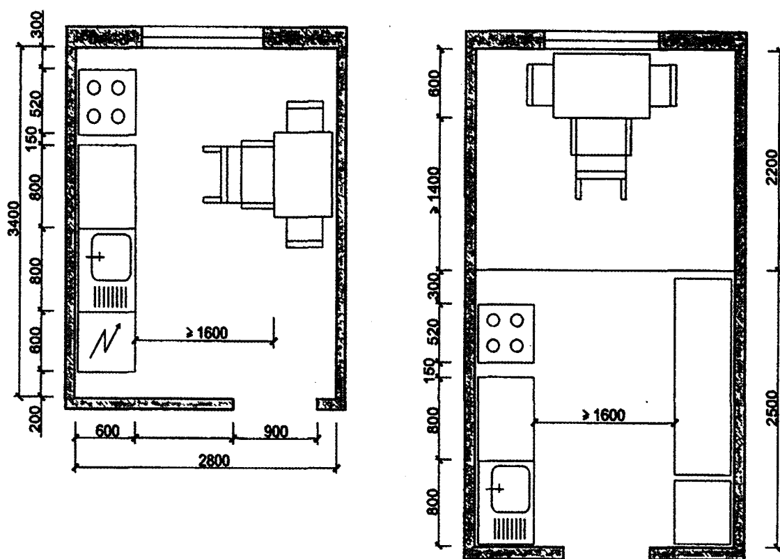
Рис. 35. Варианты кухни для жилой ячейки на 2-3 комнаты
