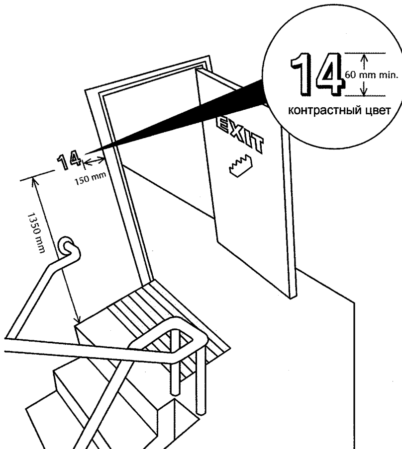
Рис. 26. Тактильная маркировка начала марша. Указатель номера этажа и знак «выход»
