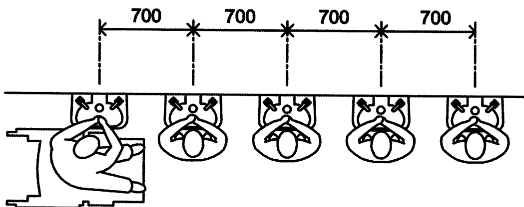
Рис. 38. Возможность подъезда к умывальнику
