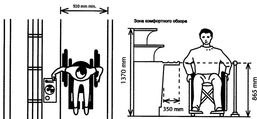
Рис. 47. Оборудование зоны обслуживания
