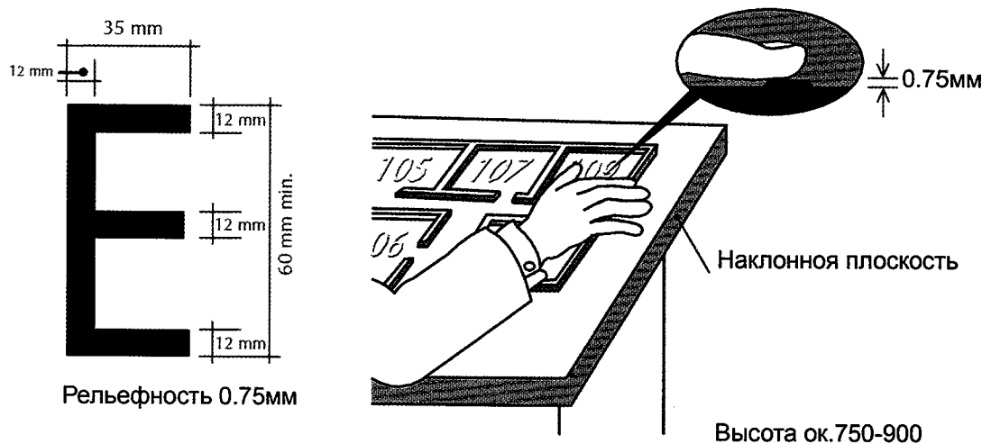
Рис 21.1 Тактильный план этажа
