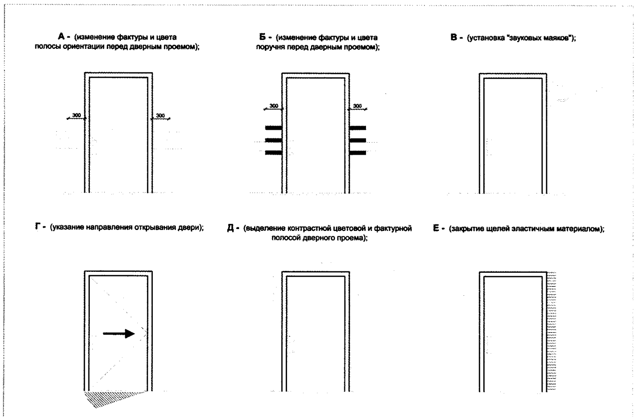
Рис. 20 Оборудование дверных проемов
