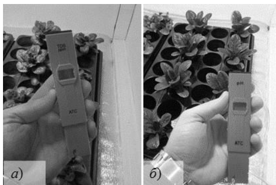
Рисунок 5 – Приборы для приготовления раствора удобрений: а) прибор для определения общего количества растворенных твердых веществ (ppm); б) pH-метр с автотемпературной компенсацией
