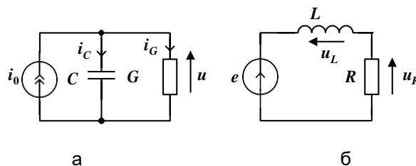
Рисунок 1 – Дуальные электрические цепи
