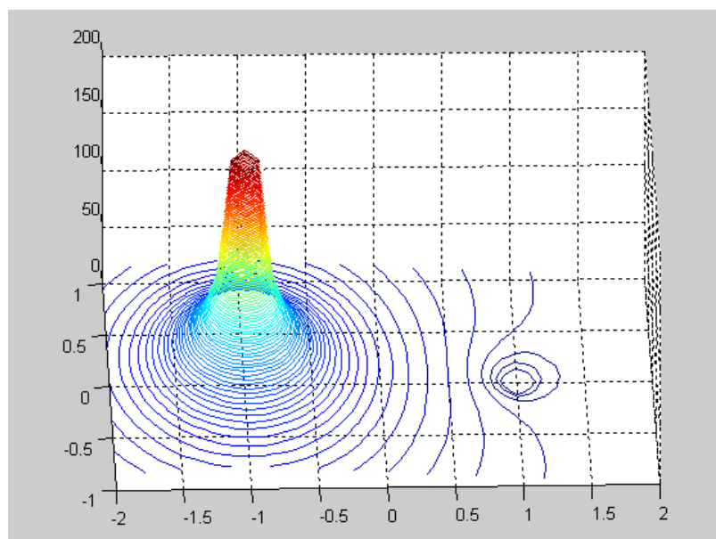
Рисунок 4 – Распределение электрического потенциала точечного заряда в трехмерном пространстве
