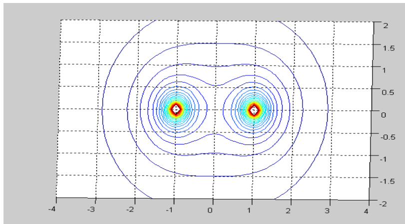
Рисунок 3 – Распределение электрического потенциала двух зарядов
