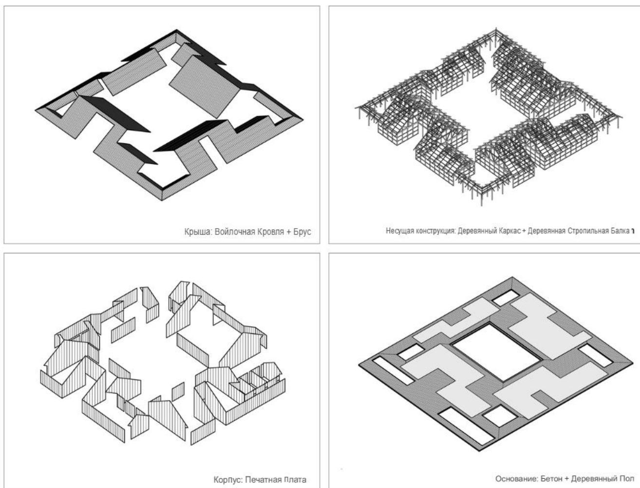
Рисунок 1. Органическая ферма в районе Тяньшань, Китай. Форма и конструкция кровли
