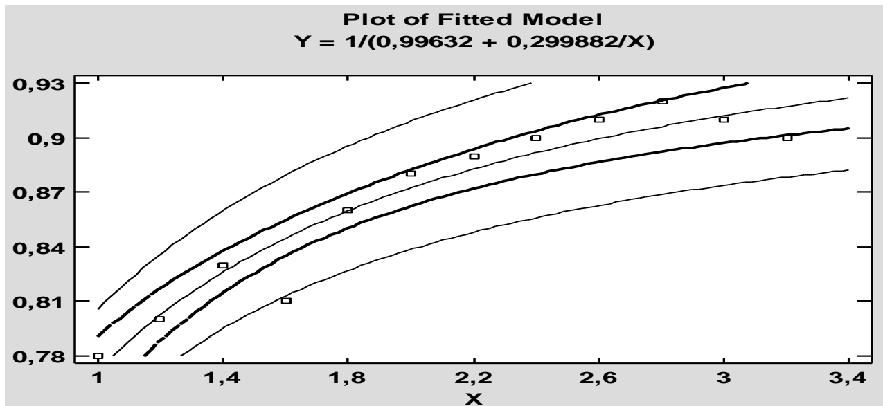
Рисунок 1 – Изменение типового показателя ( y , усл.ед.) при изменении величины зазора между рабочими органами шелушительной машины ( x , мм).
