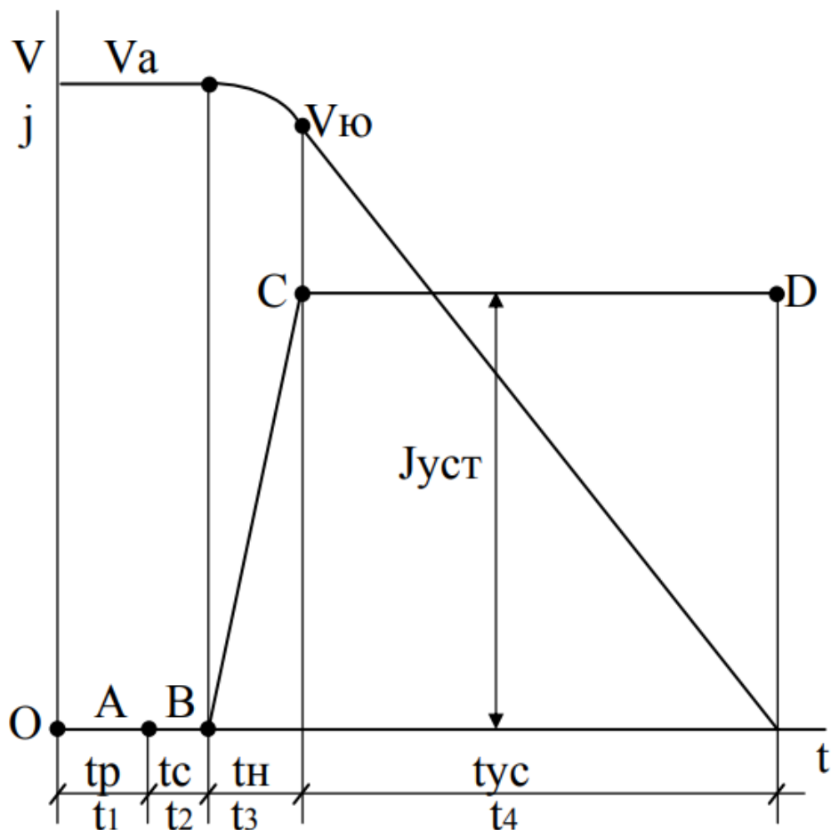
Рисунок 1 – Диаграмма снижения скорости автомобиля при торможении
