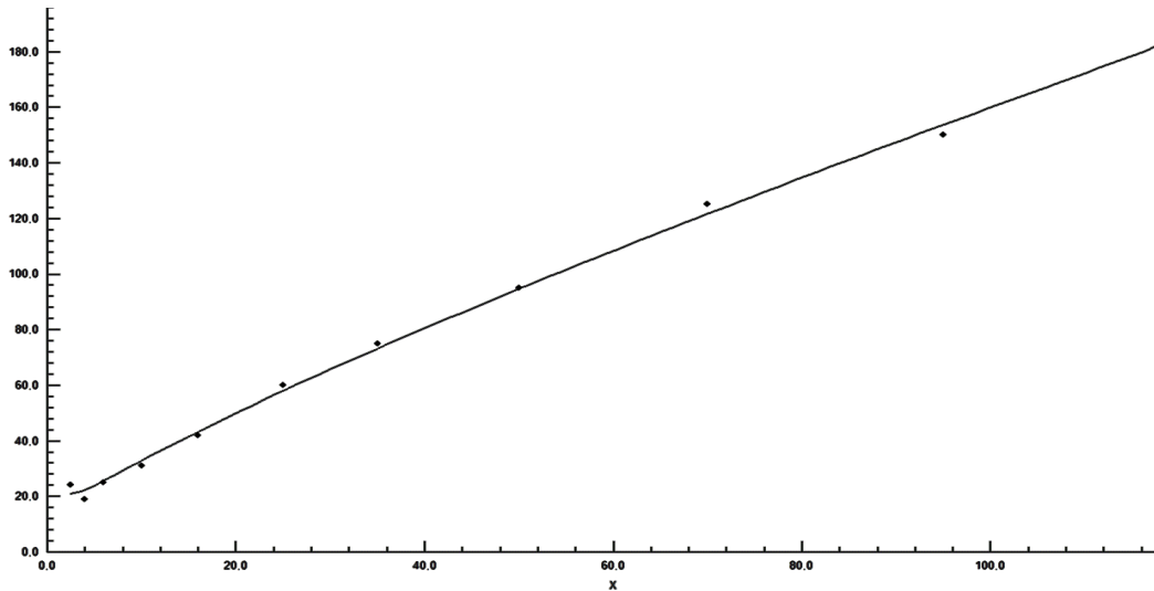
Рисунок 2 – Изменение токовой нагрузки при выборе провода двужильного с площадью сечения токопроводящей жилы 2.5...120 мм 2 проложенного в одной трубе, А Коэффициент детерминации выявленной зависимости составляет 99,82% > 95%.
