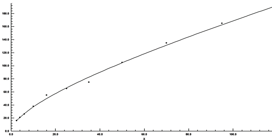
Рисунок 2 – Изменение токовой нагрузки при выборе провода трёхжильного с площадью сечения токопроводящей жилы 2.5...120 мм 2 проложенного в одной трубе, А
