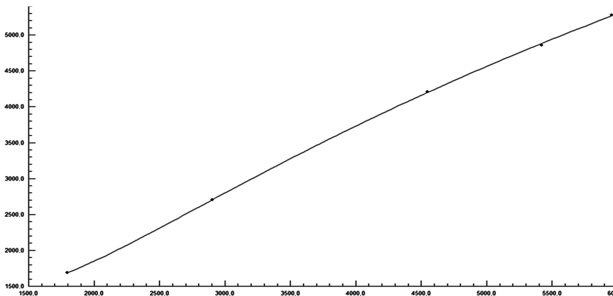
Рисунок 1 – Изменение активной мощности на выходе трансформатора при изменяющейся однофазной нагрузке, Вт
