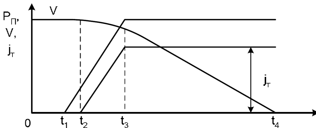
Рисунок 1 - Диаграмма торможения ТС: V – скорость ТС, км/ч; P_{П} – усилие на педали, Н; j_T – замедление ТС, м/с 2 ; t_1 – время реакции водителя, с; t_2 – время запаздывания срабатывания тормозной системы, с.; t_3 – время нарастания замедления с.; t_4 – время торможения ТС, с.
