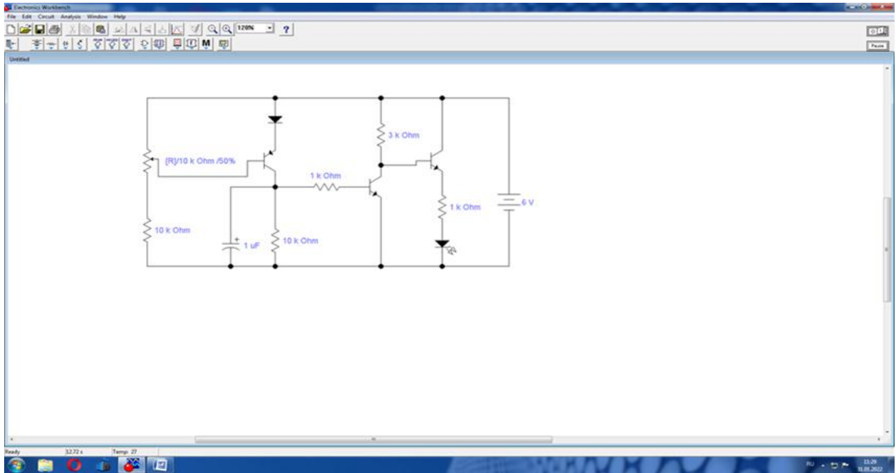
Рисунок 1 – Модель схемы световой сигнализации температуры
