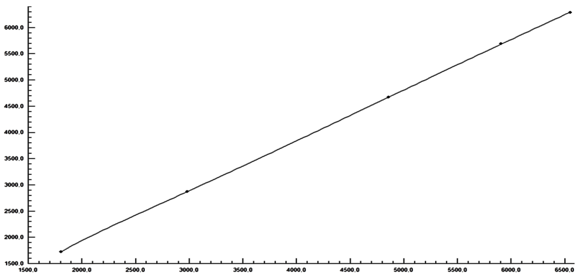
Рисунок 3 – Изменение активной мощности на выходе трансформатора при переменной однофазной активной нагрузке, Вт
