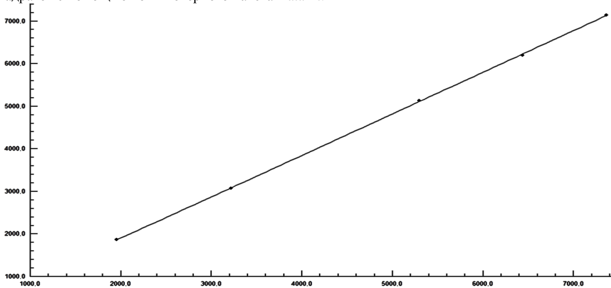
Рисунок 2 – Изменение активной мощности на выходе трансформатора при переменной несимметричной трёхфазной активной нагрузке, Вт
