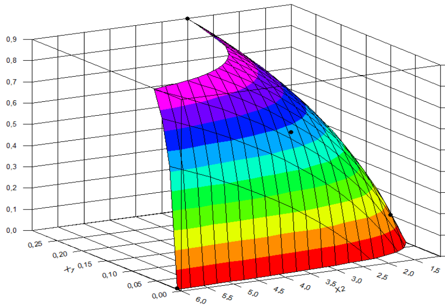
Рисунок 5 – Прогнозируемые области интенсивности отказов ( y, ч^{-1} ) в зависимости от интенсивности отказа одного электрорадиоэлемента ( x_1, ч^{-1} ) и их количества ( x_2, шт. )
