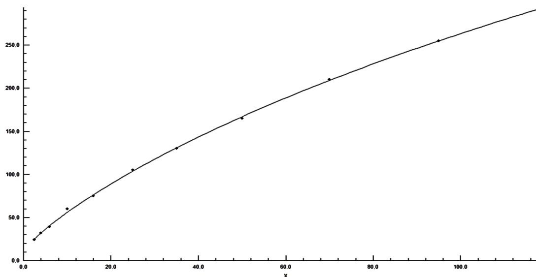
Рисунок 1 – Изменение токовой нагрузки при выборе провода с площадью сечения токопроводящей жилы 2.5...120 мм 2 проложенного открыто, А
