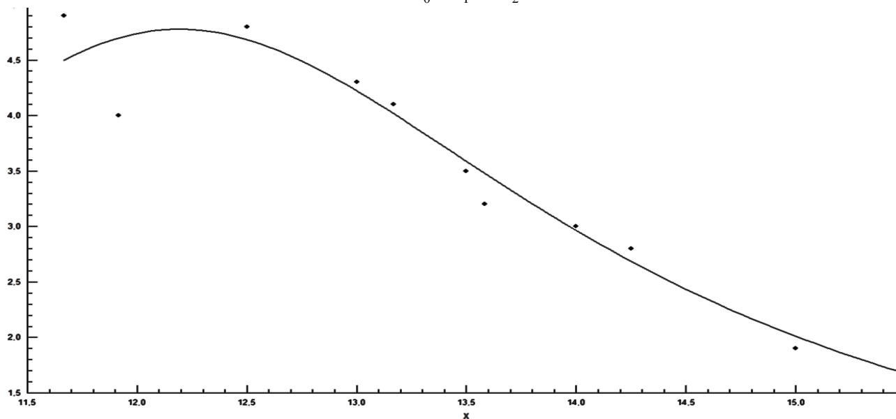
Рисунок 1 – Изменение вырабатываемой мощности солнечным модулем с круглым концентратором во временном интервале 11:40 – 15:30 ( t, ч )
