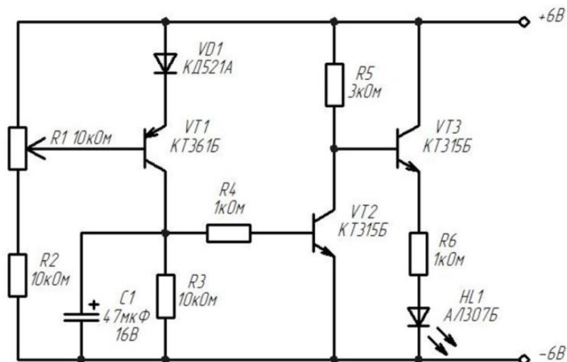
Рисунок 2 – Принципиальная схема световой сигнализации датчика температуры
