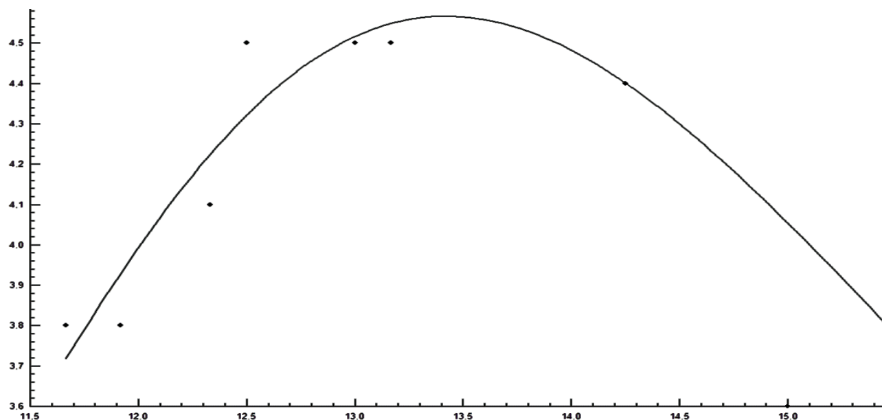
Рисунок 2 – Изменение вырабатываемой мощности солнечным модулем с шестиугольным концентратором во временном интервале 11:40 – 15:30 ( t, ч )
